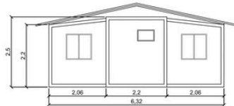
VISTA TRASERA
